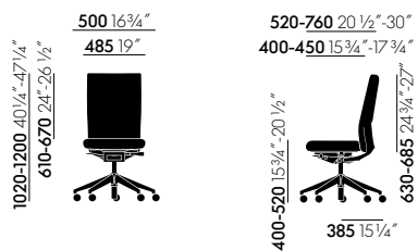
ID Soft L ohne Armlehnen
