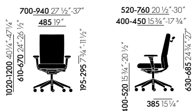
ID Soft L mit 3D-Armlehnen und Kleiderbügel
