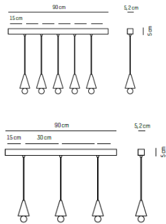
Platine linéaire
