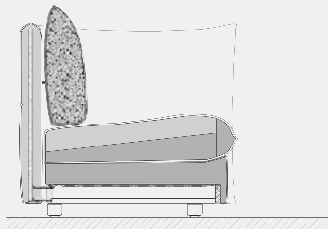
Schnitt durch den Polsteraufbau
