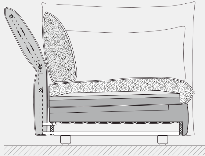
Schnitt durch den Polsteraufbau
