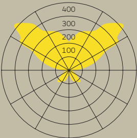
kido 50/56 125lm/W@4000K
