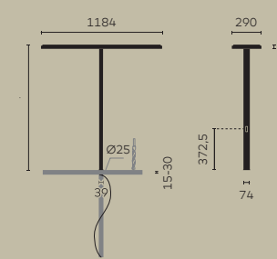
kido Tischaufbauleuchte Doppelkopf asymmetrisch
