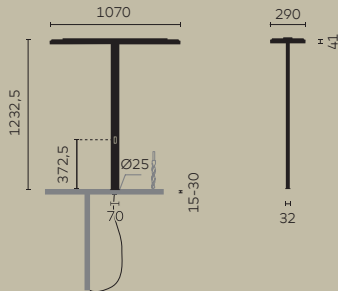
kido Tischaufbauleuchte
