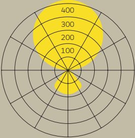
kido 32 140lm/W@4000K
